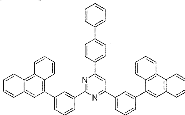
(HB-1)
