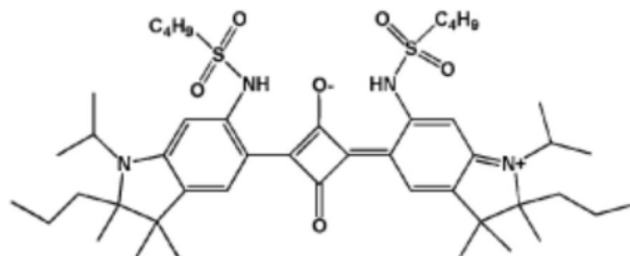
化合物 1
