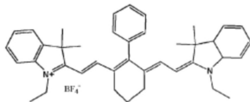
化合物 4
