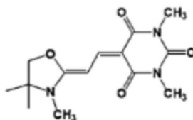
化合物 3
