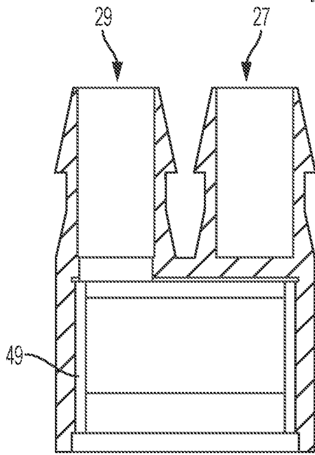
SECTION D-D
