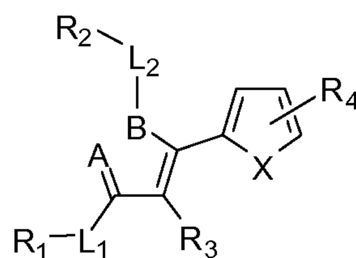
Formula (D);
