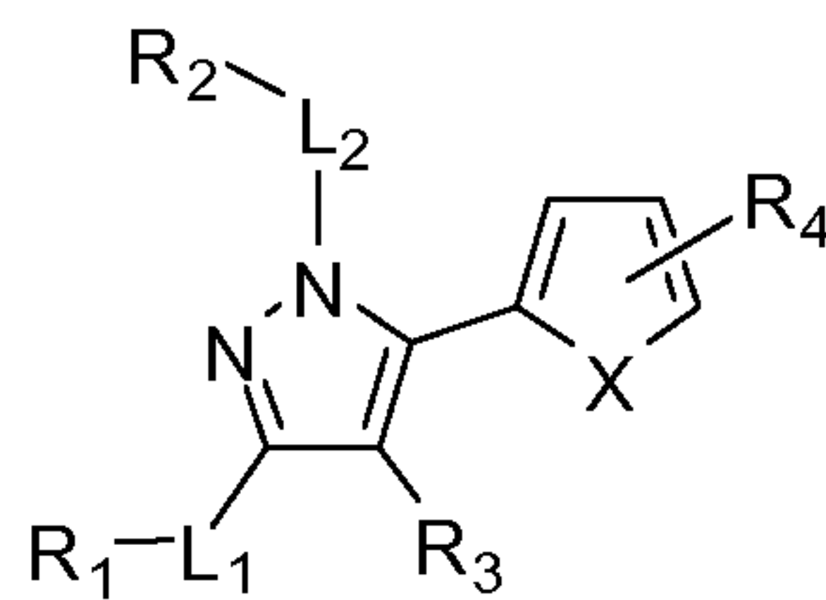
Formula (VI);
