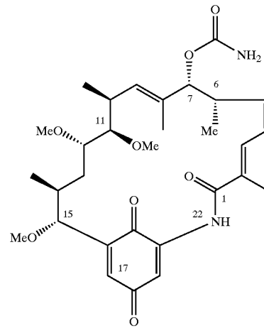
Macbecin I
