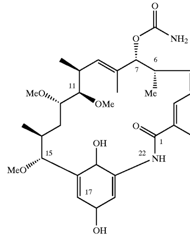
Macbecin II
