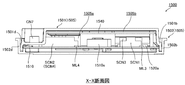
X-X断面图
