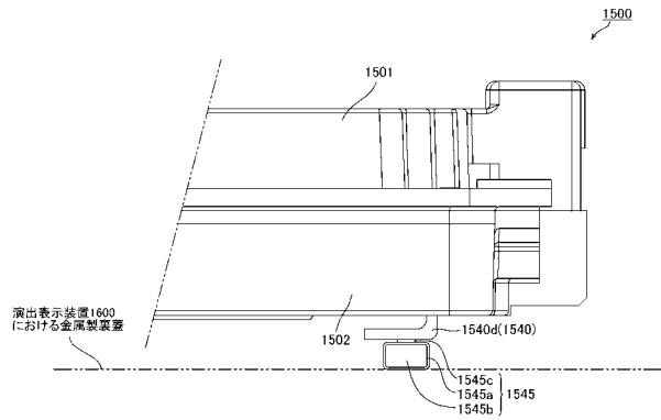
A矢視図
