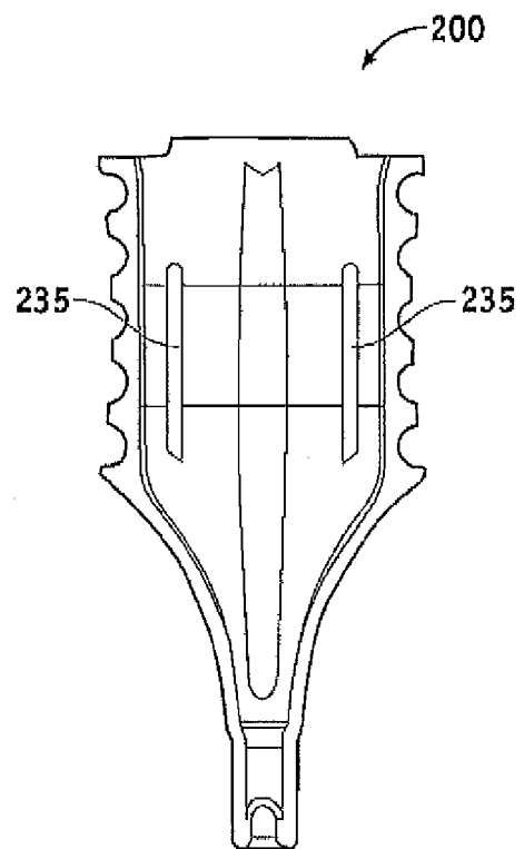
FIG. 23B SECTION B-B
