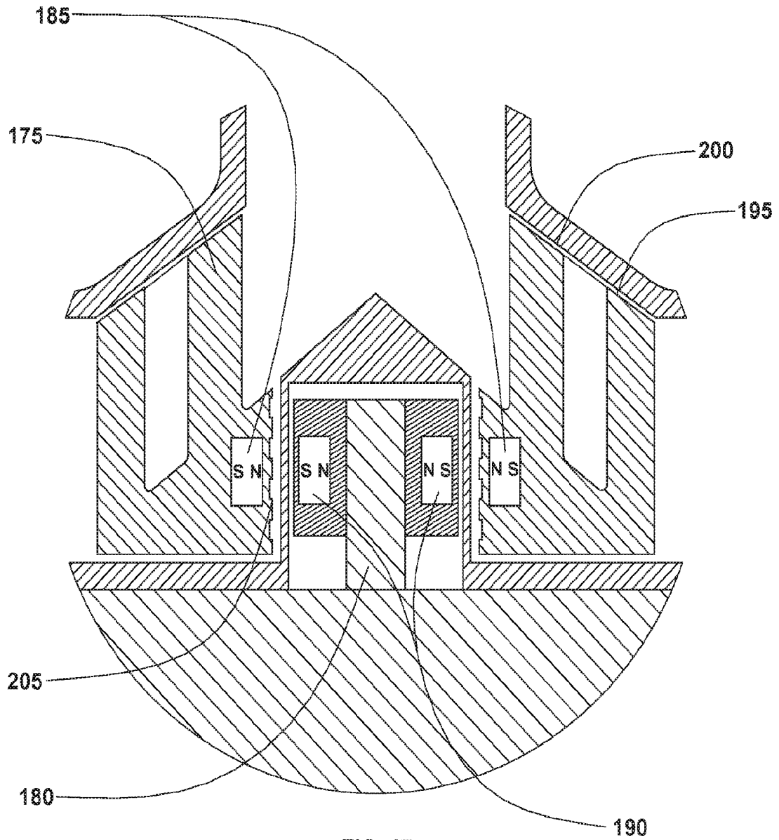
FIG. 17 (DETAIL E)
