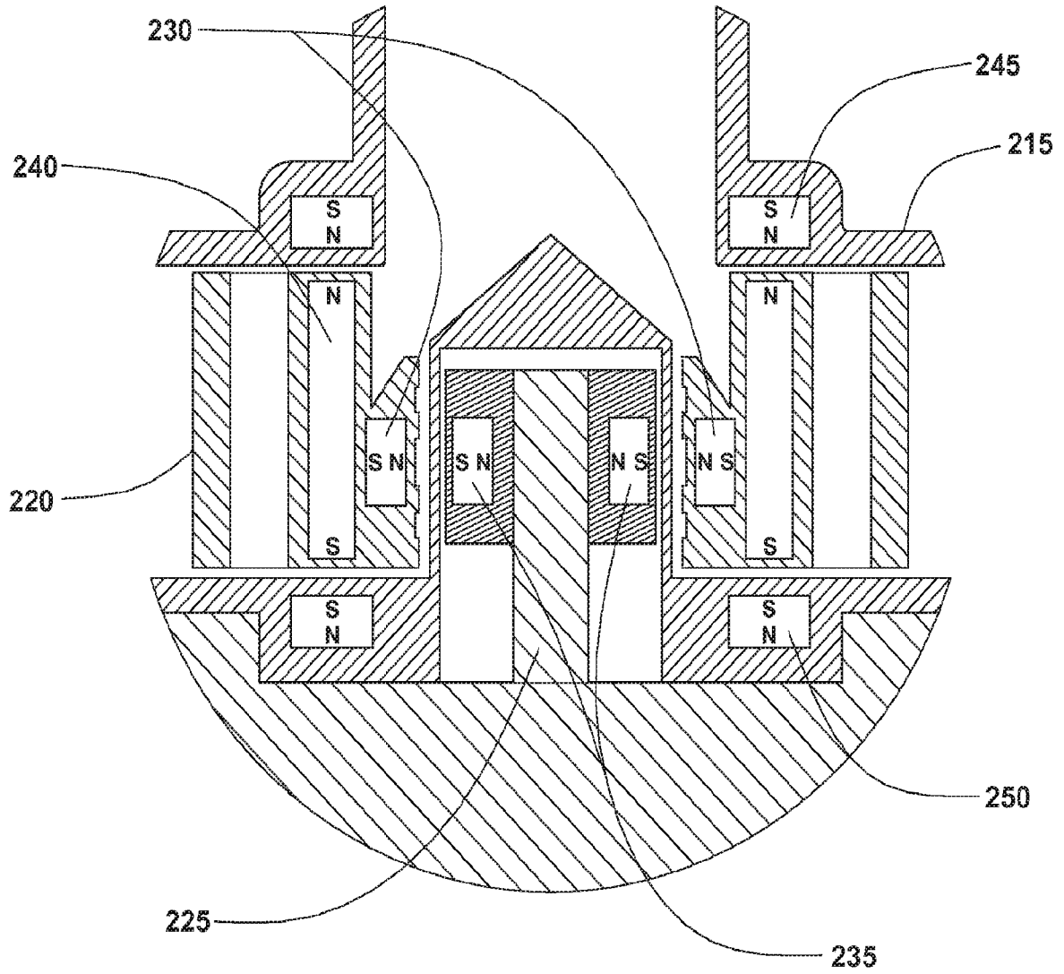
FIG. 20 (DETAIL H)
