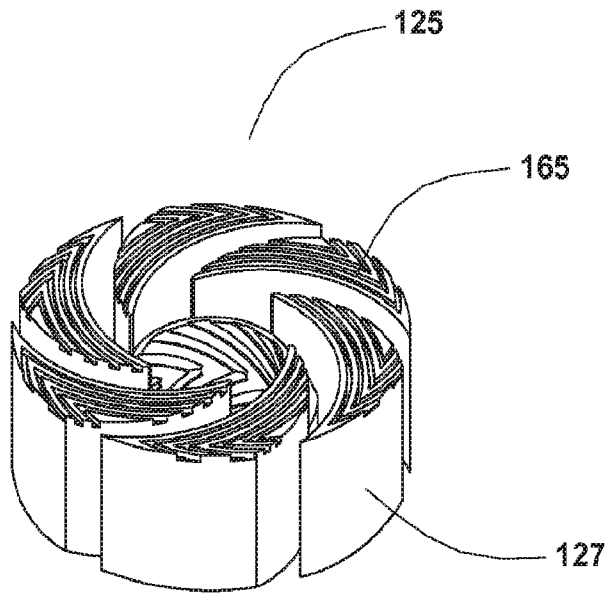
FIG. 14A
