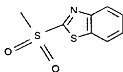
2-benzothiazolsulfonyl
