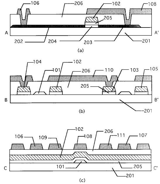
実施例1断面図
