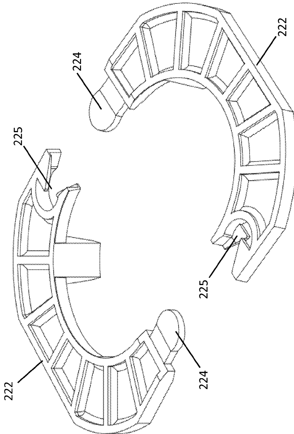
FIG. 7B
