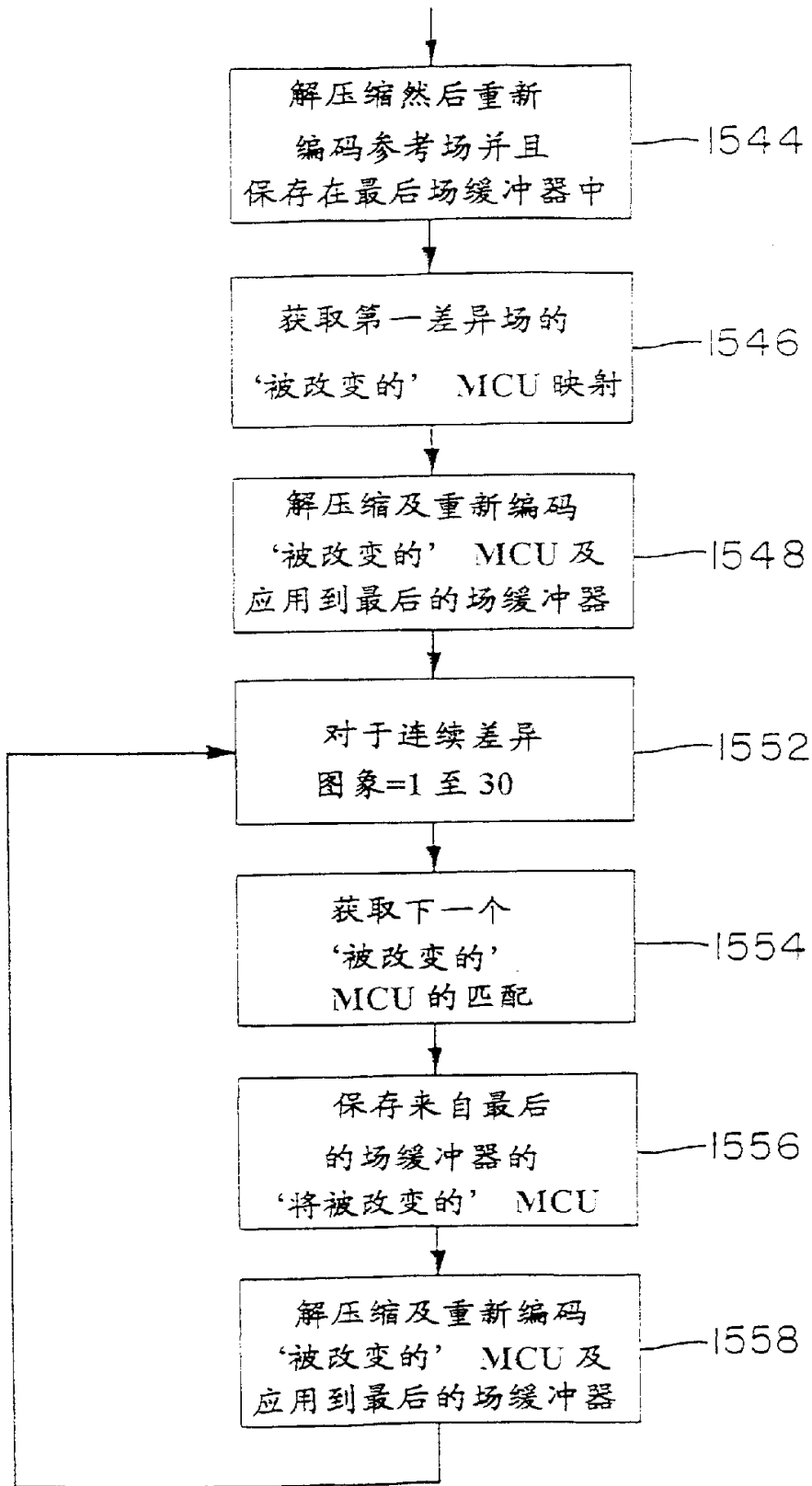
图 66 建立后向历史缓冲器
