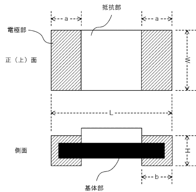
チップ抵抗 (10Ω~10MΩ) サイズ表
