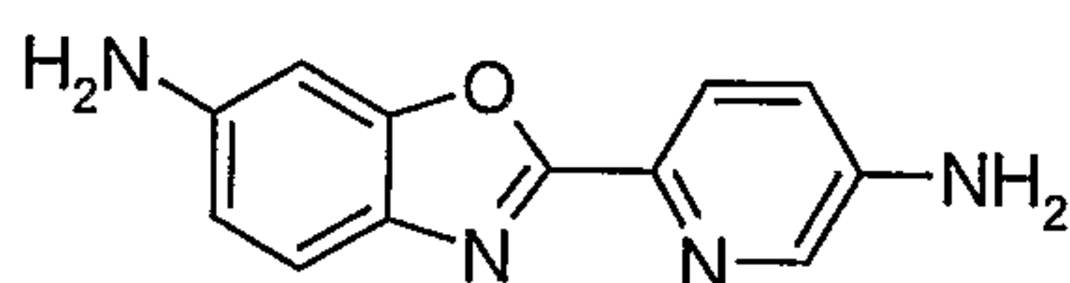
2-(5-aminopyridin-2-yl)-1,3-benzoxazol-6-amine
