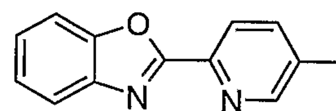
2-(5-methylpyridin-2-yl)-1,3-benzoxazole
