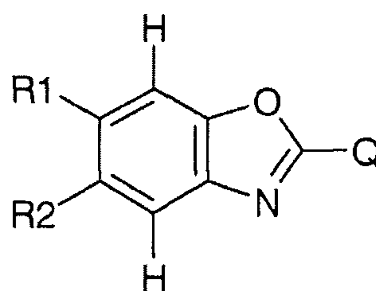
(Ia)
