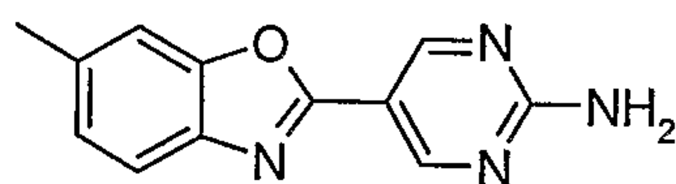
5-(6-methyl-1,3-benzoxazol-2-yl)pyrimidin-2-amine
