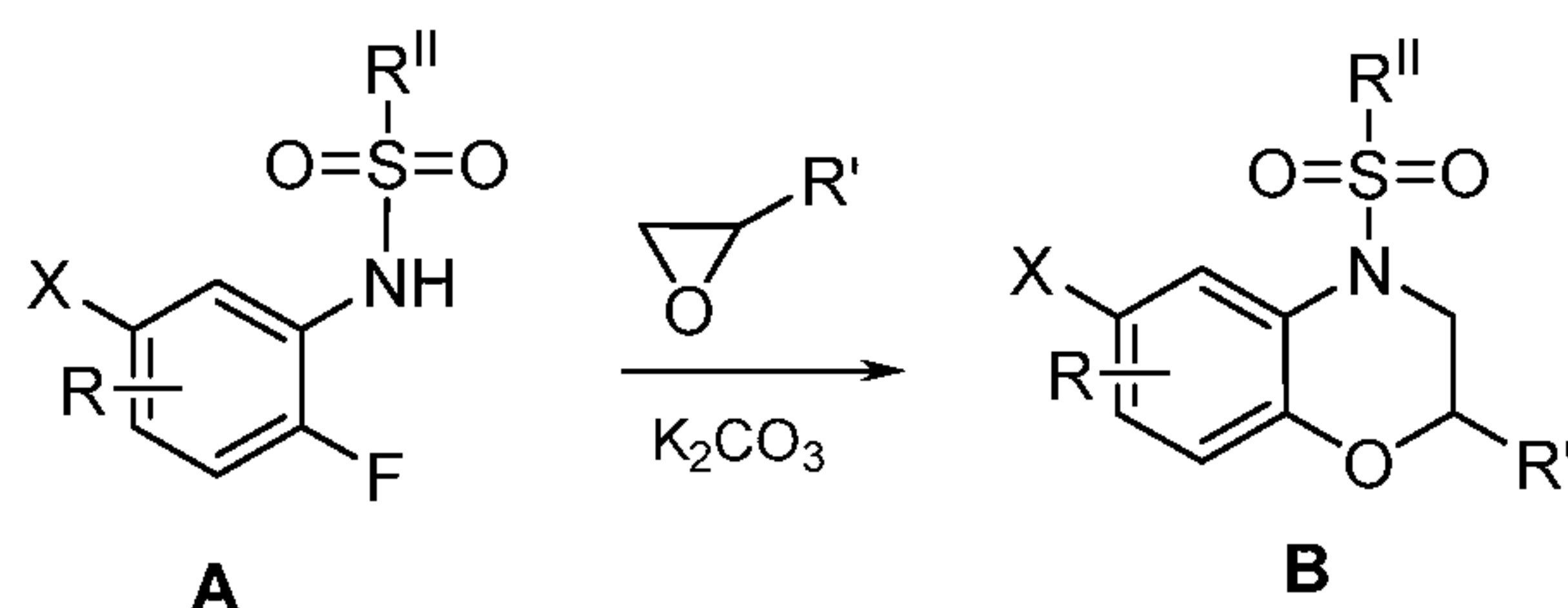
SCHEME 16.
