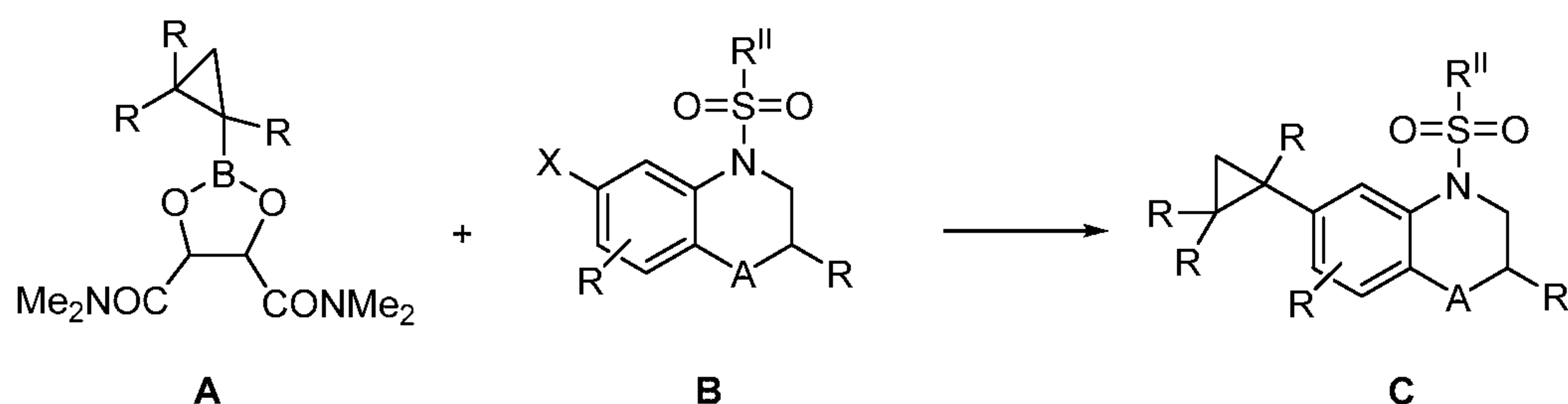
SCHEME 14.
