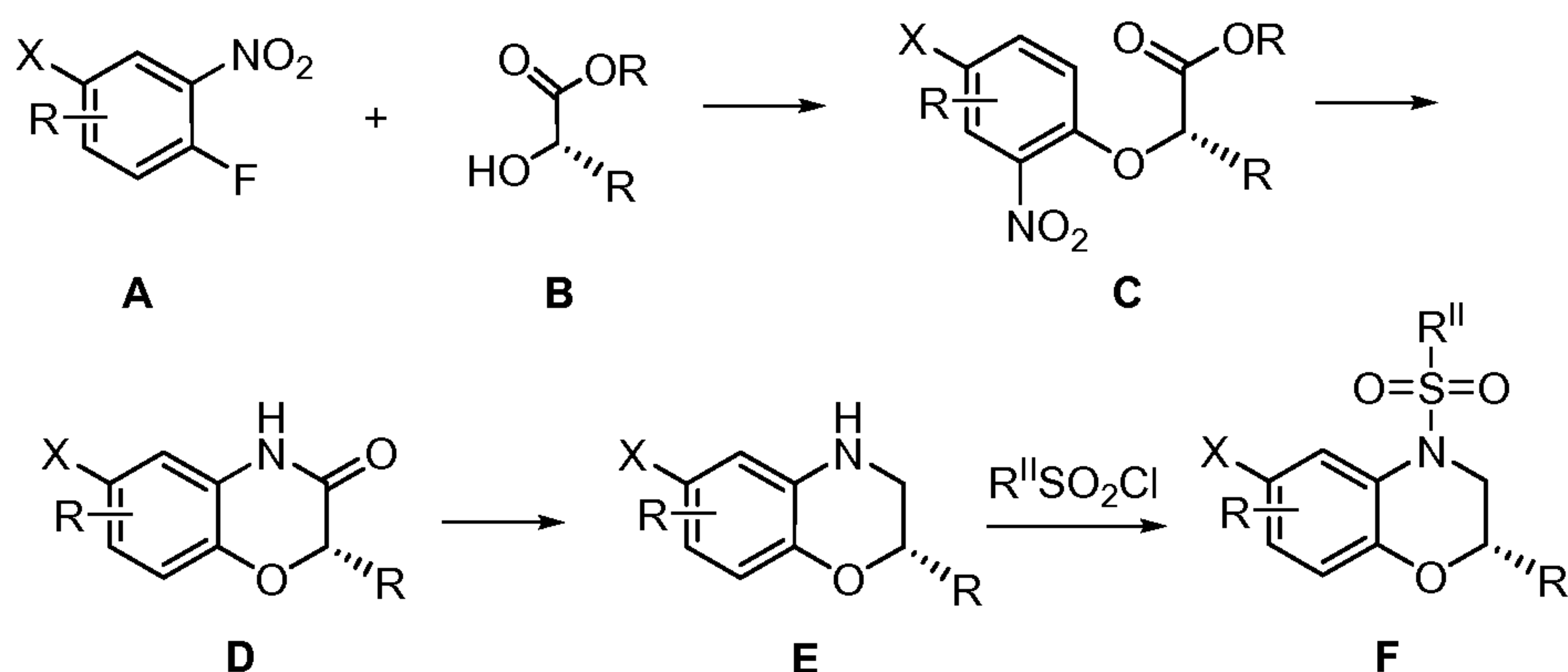
SCHEME 17.
