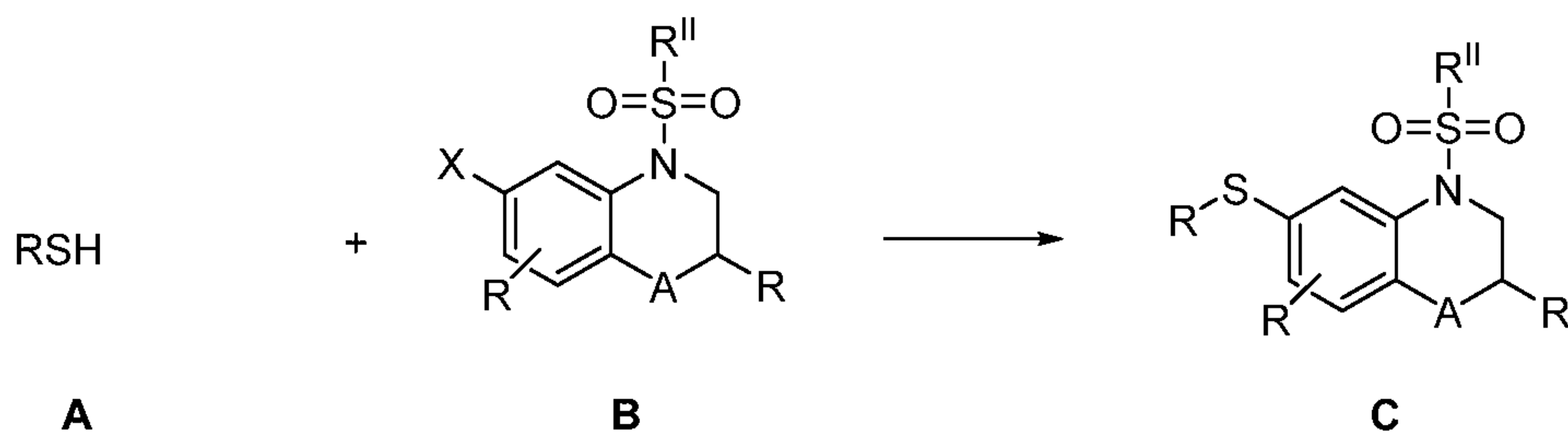
SCHEME 19.
