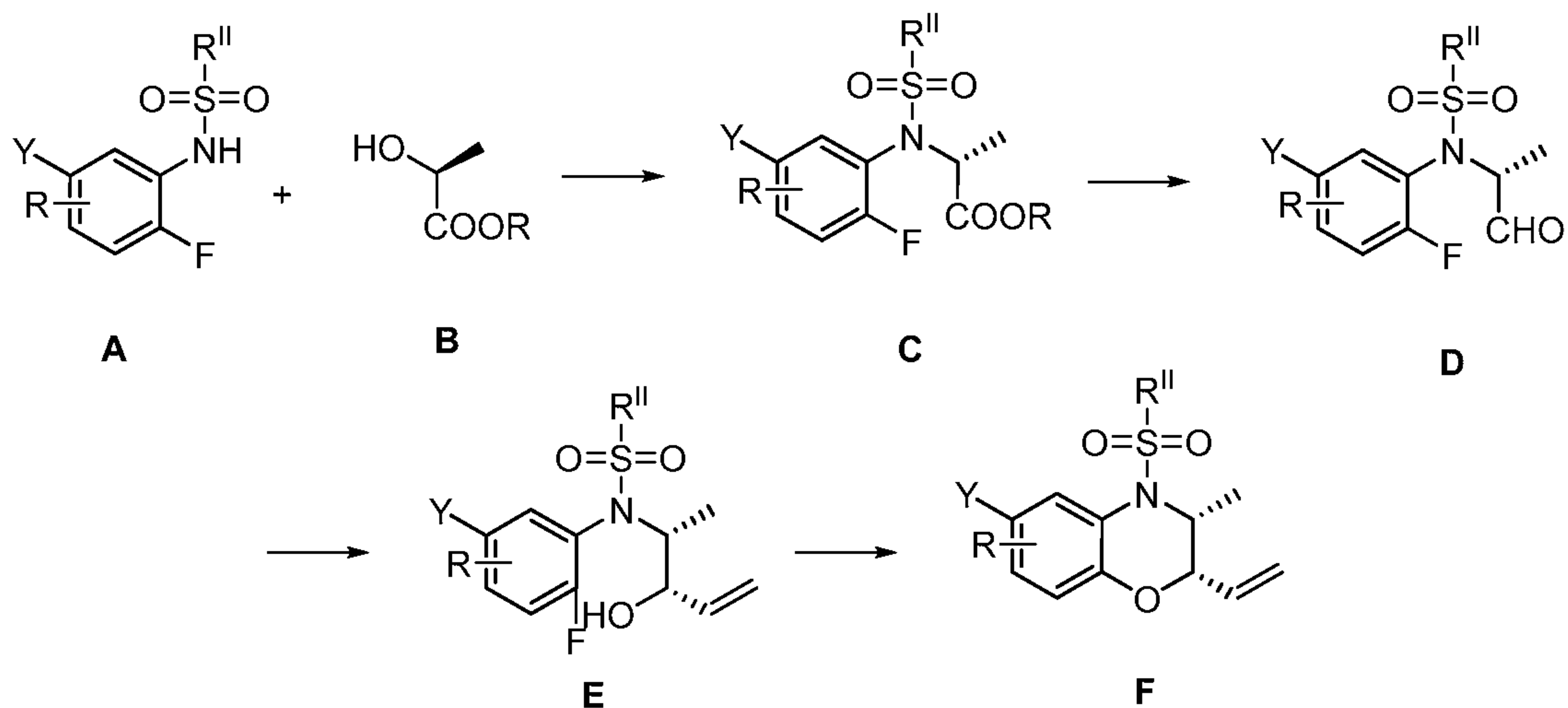
SCHEME 18.
