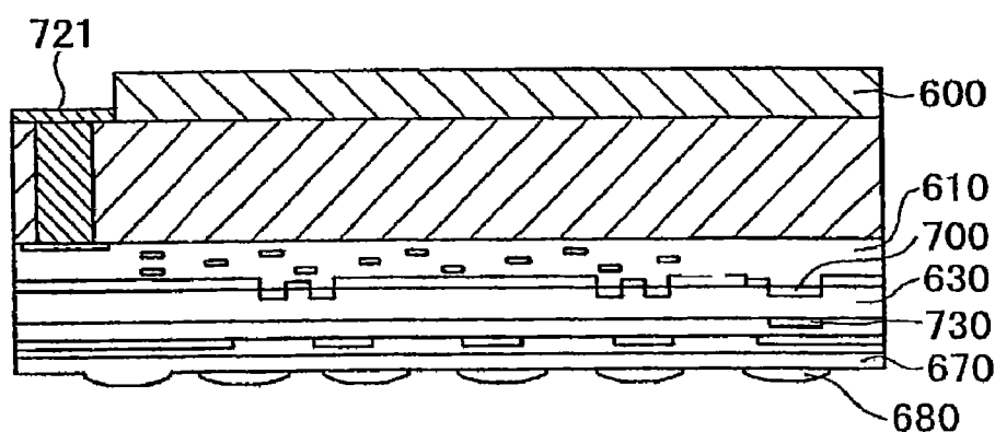
FIG. 10J
