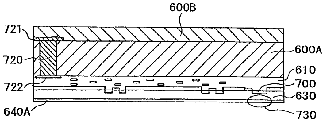
FIG. 9G
