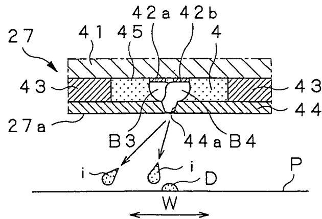
FIG. 16C
