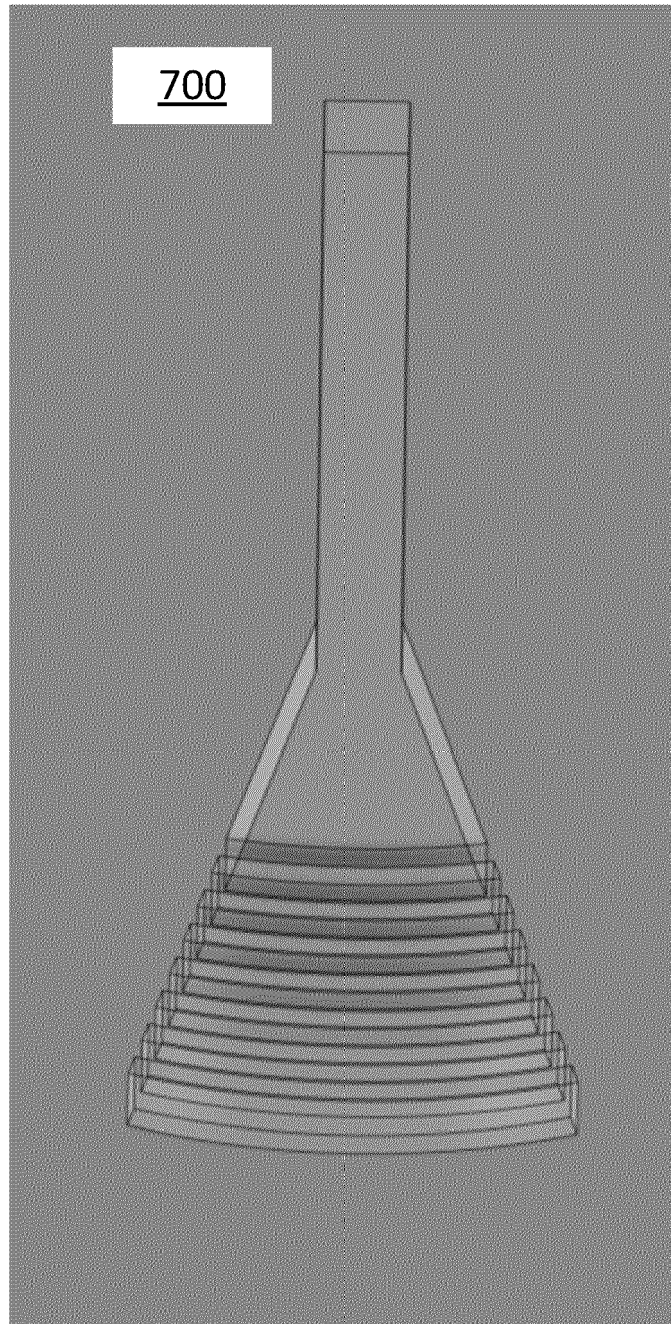
FIG. 7 Waveguide
