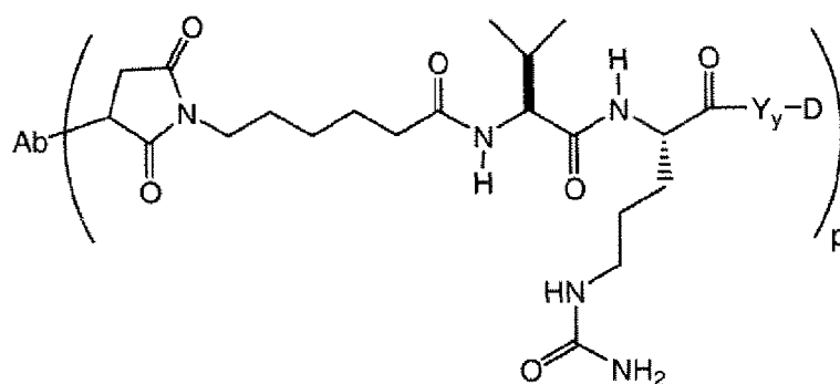
MC-val-cit
