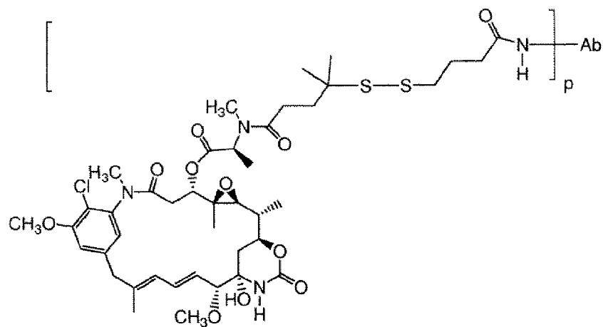
Ab-SPDB-DM4
