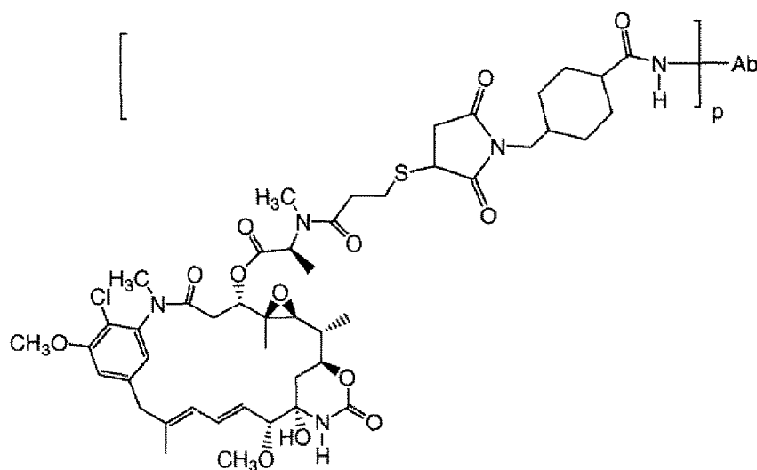
Ab-SPDB-DM4
