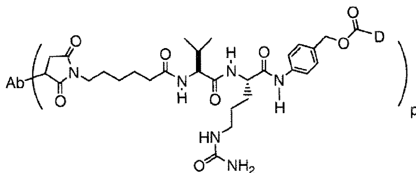
MC-val-cit-PAB
