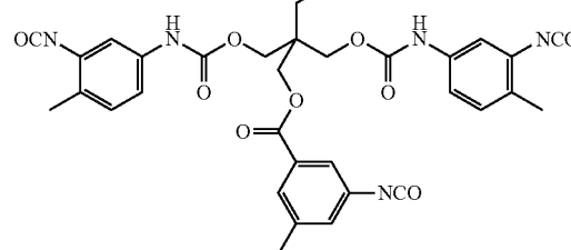
DESMODUR L75
