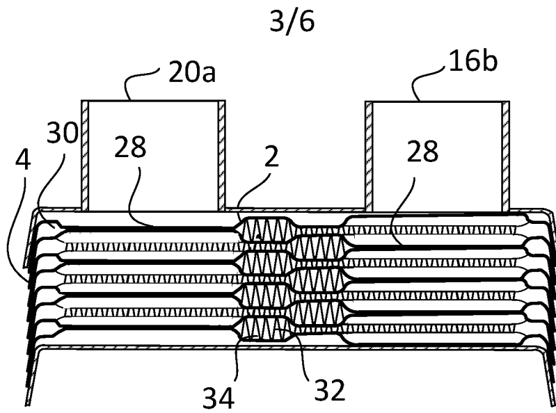
Fig. 5 (V – V)
