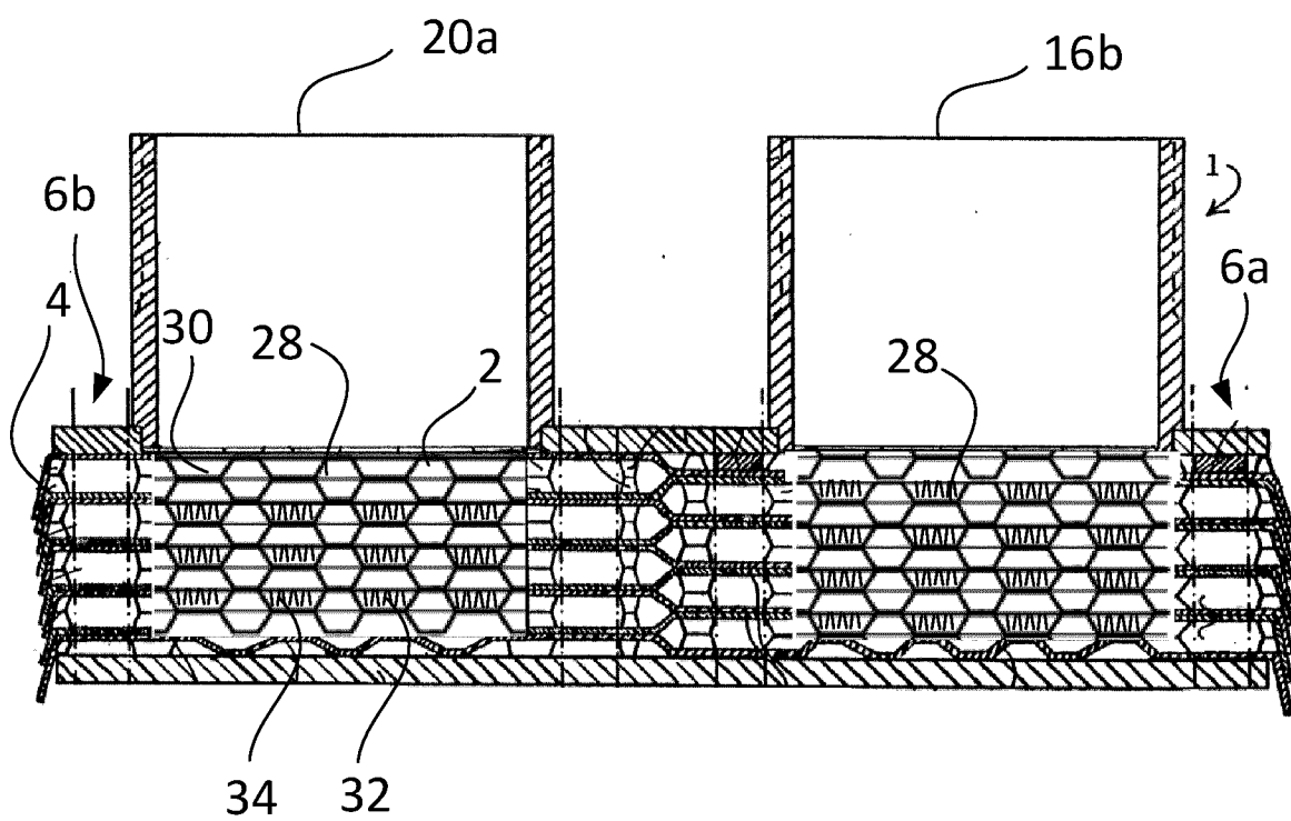
Fig. 6 (V – V)
