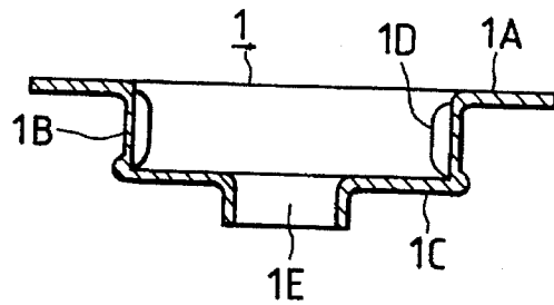
FIG. 2E
