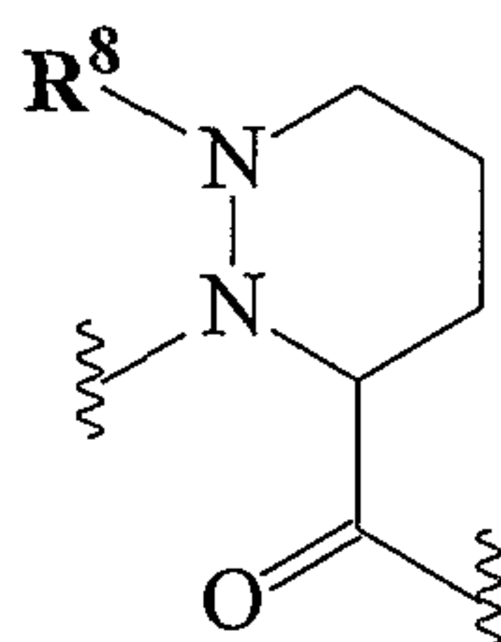
IIg
