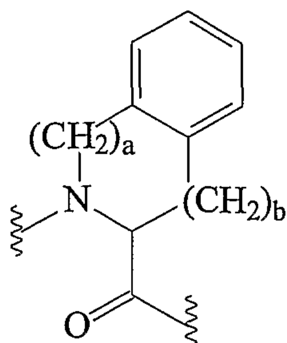
IIh
