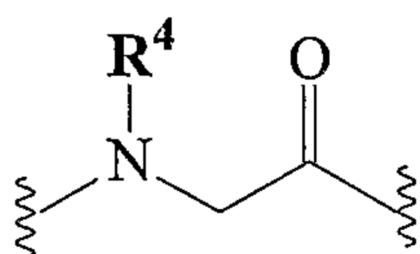
IIb
