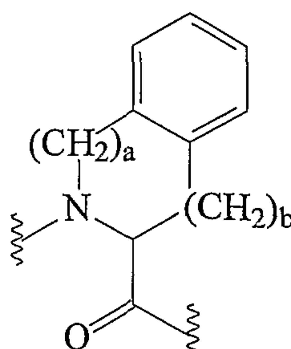
IIh
