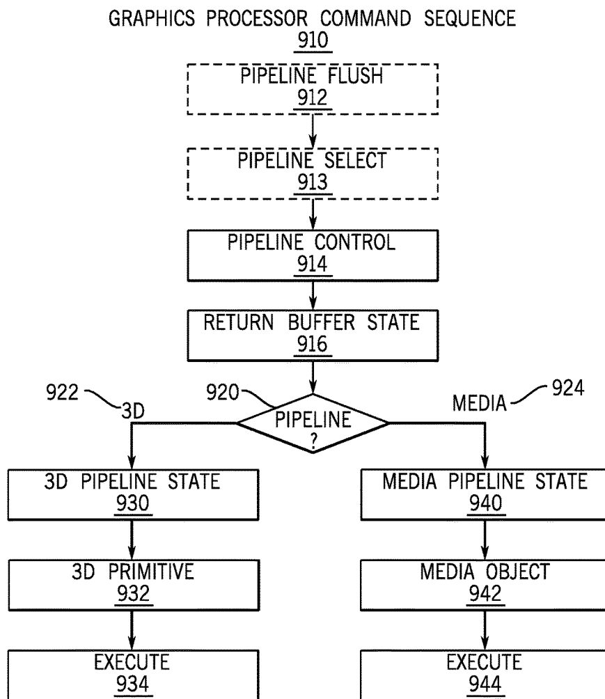
FIG. 14B
