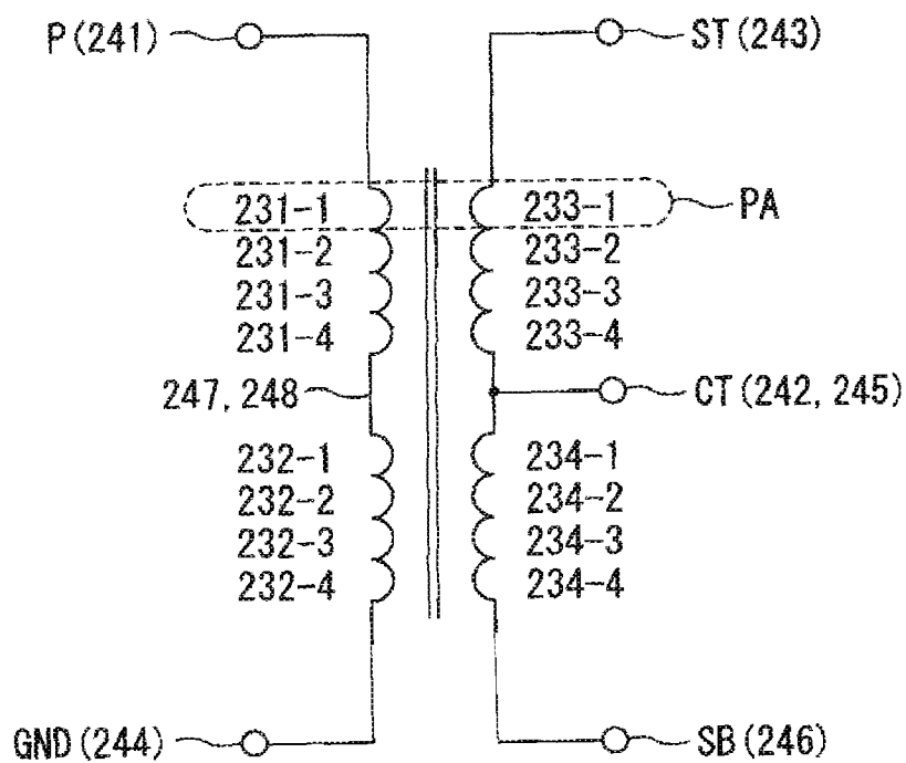
FIG.13A
