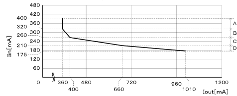
(b) TA点の入力電流 I_{in} 及びTB点の出力電流 I_{out}
