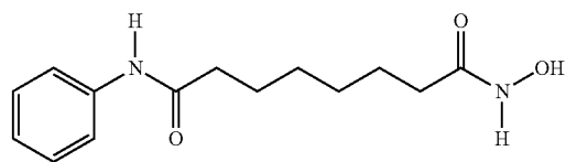
Vorinostat
