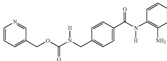
Entinostat
