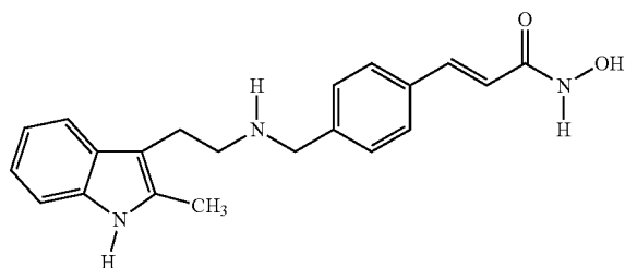
Panobinostat
