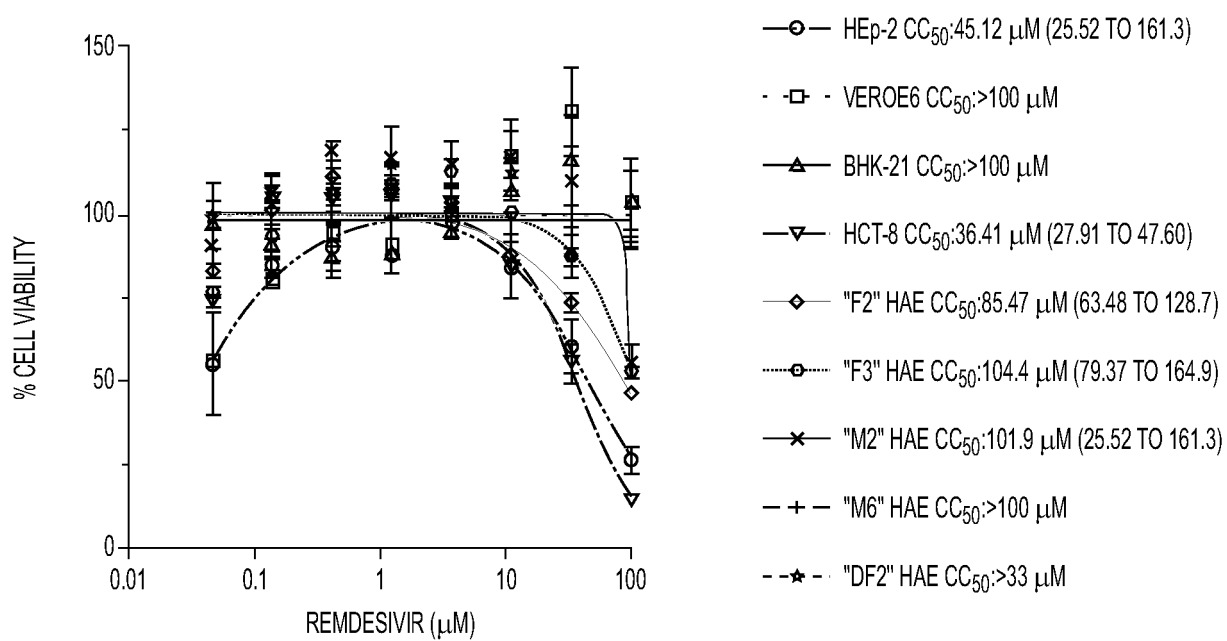
FIG. 1e
