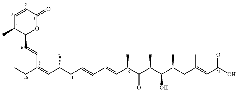
Leptomycin B
