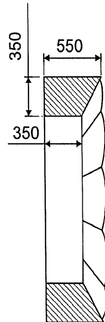
Section A-A
