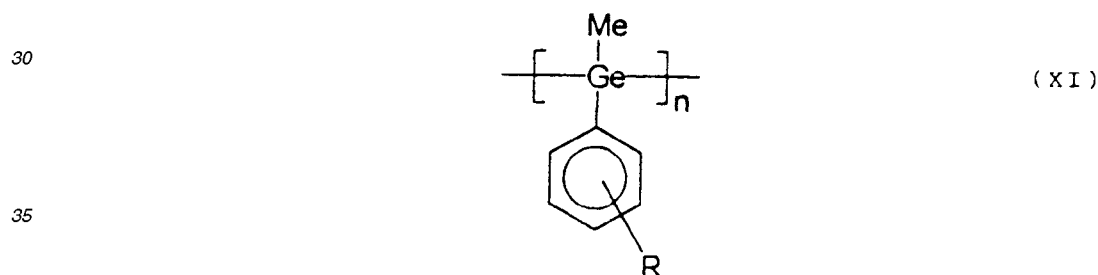
polygermane (XI)
