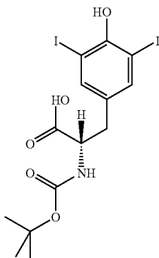
N-tert-butylloxycarbonyl-3,5-diiodo-L-tyrosine
