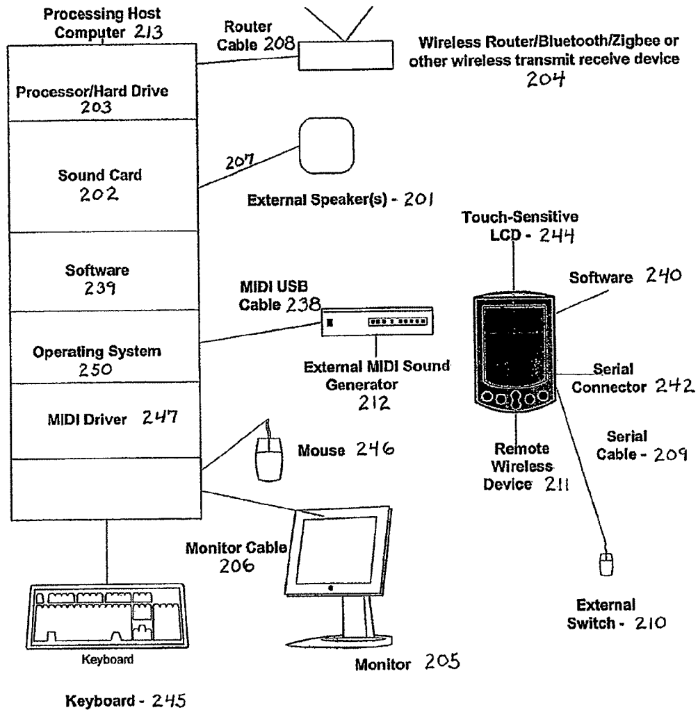
Fig. 1B- Schematic
