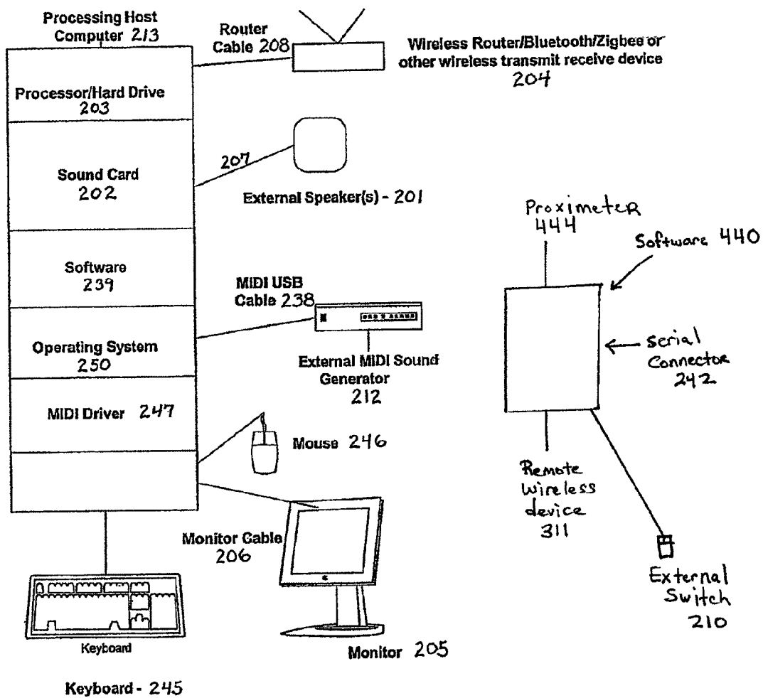
Fig. 1E Schematic
