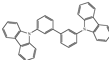
H7
