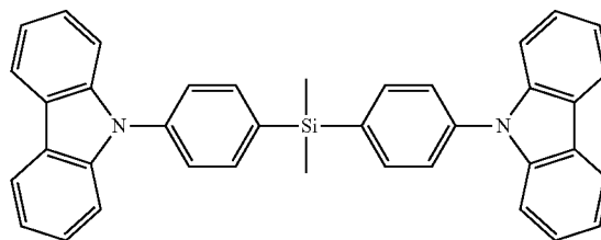
H4
