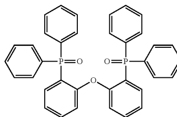
H7
