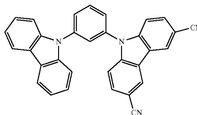
H19
