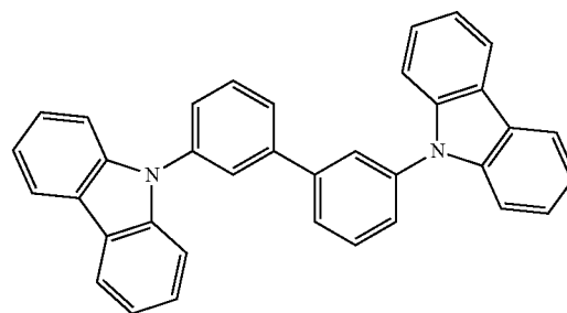
H7
