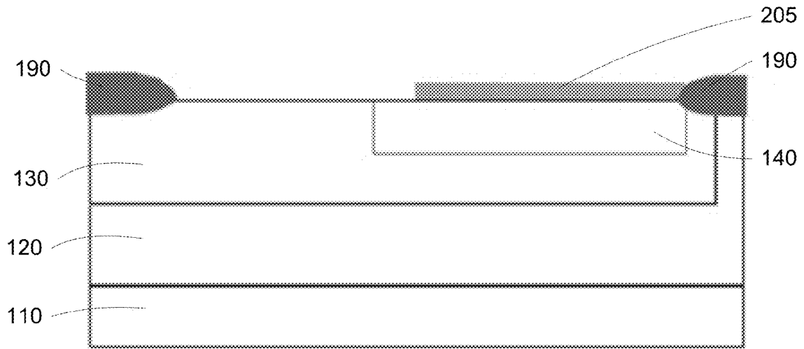
FIG. 14E
