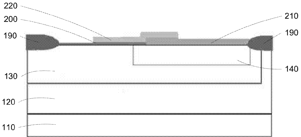
FIG. 14G
