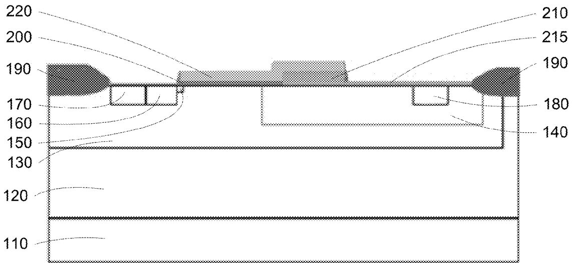
FIG. 14H
