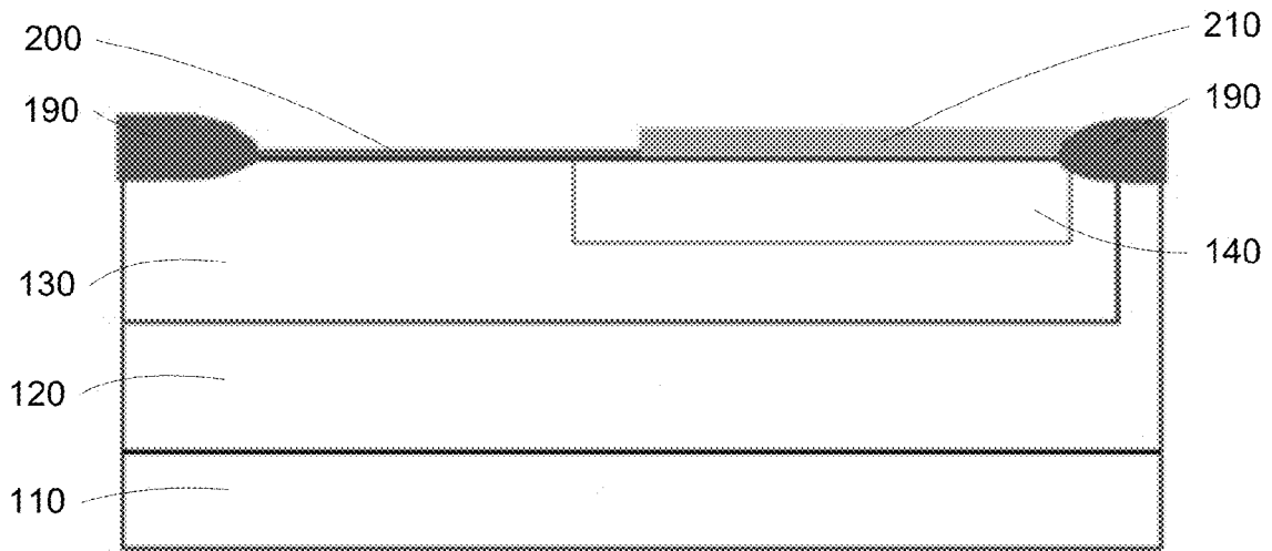
FIG. 14F
