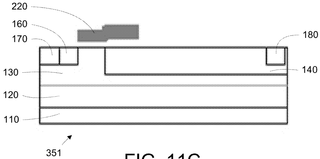
FIG. 11C
