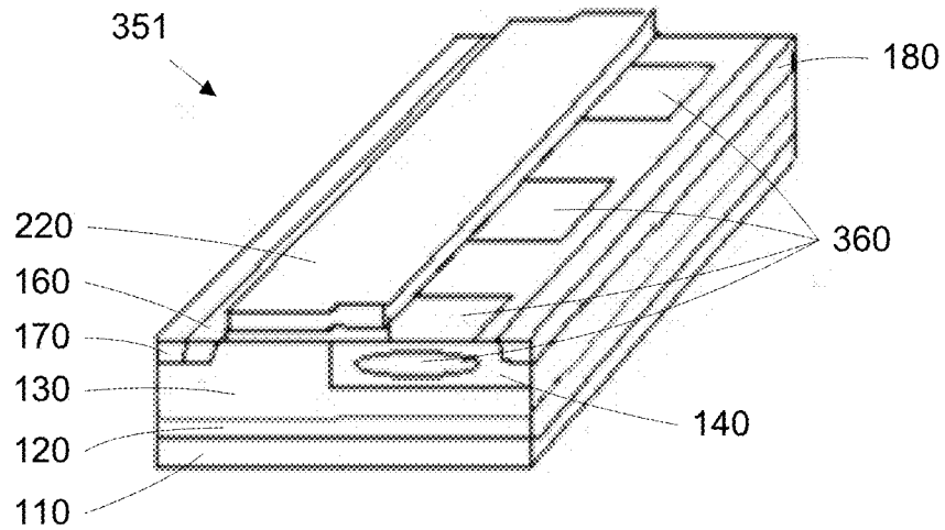
FIG. 11A
