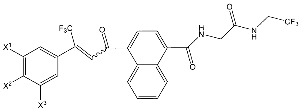
(IIA)
