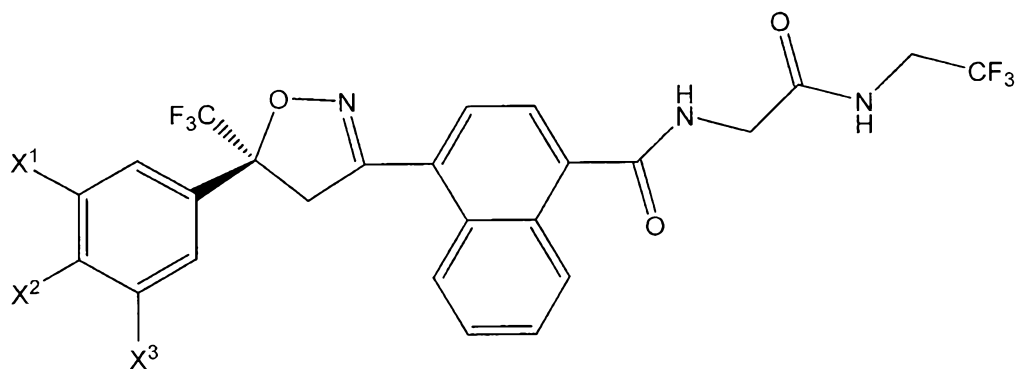
(S)-IA
