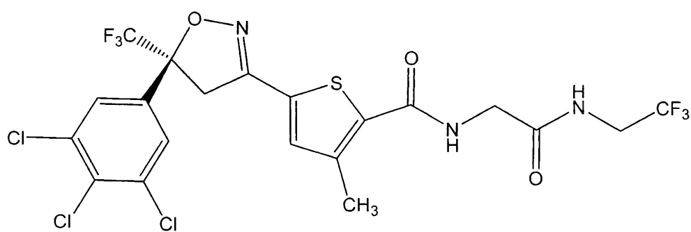
lotilaner
