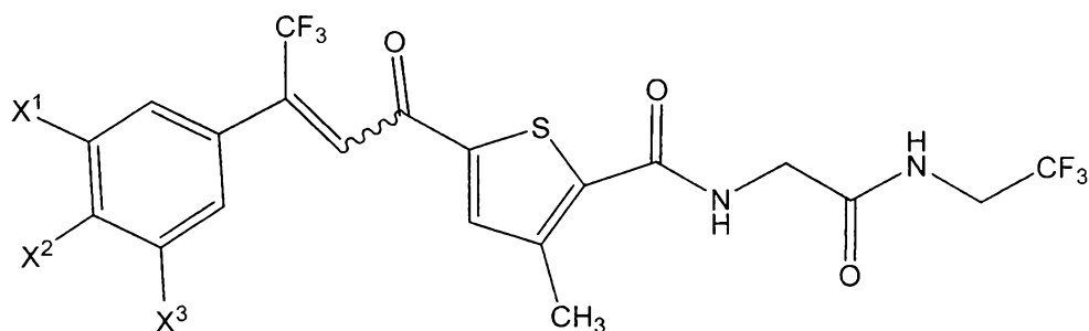
(IID)
