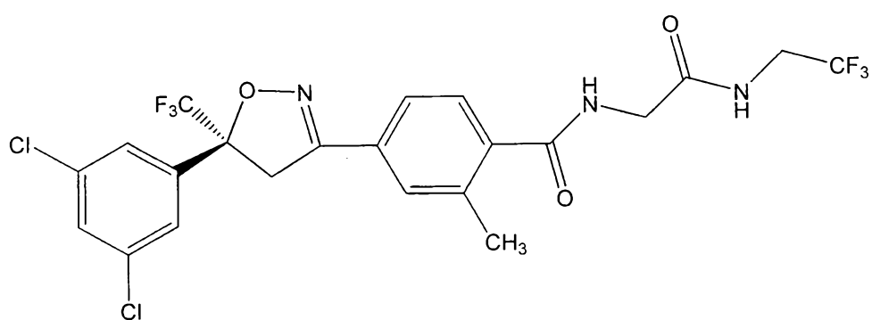
(S)-fluralaner
