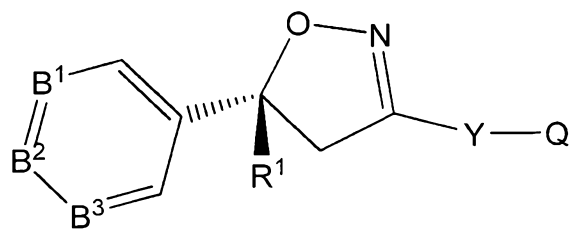
(R)-I
