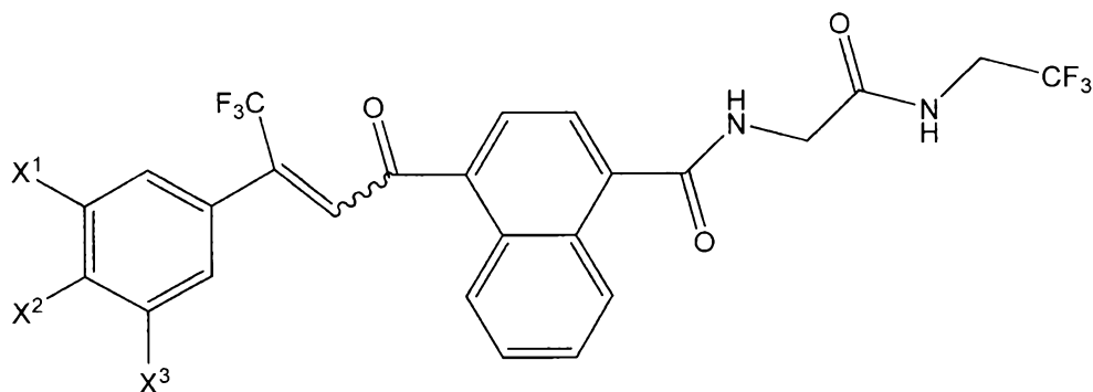
(IIA)
