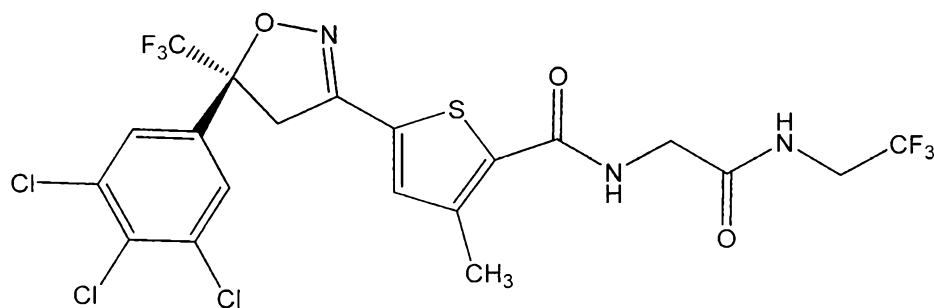
Lotilaner
