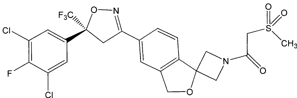
Fluralaner
