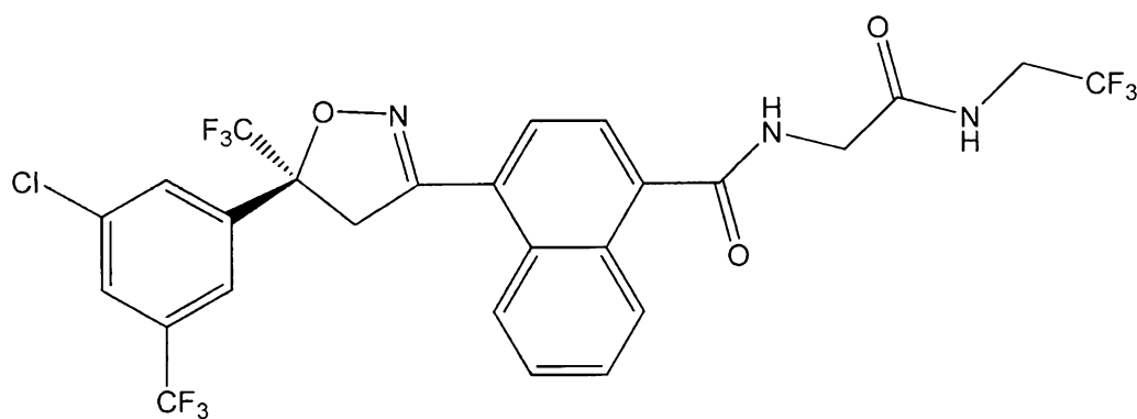
( S )-afoxolaner
