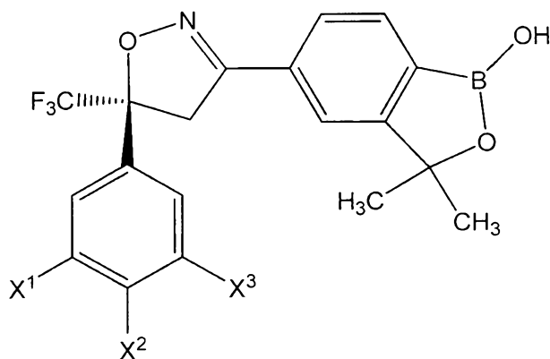
(S)-IE
