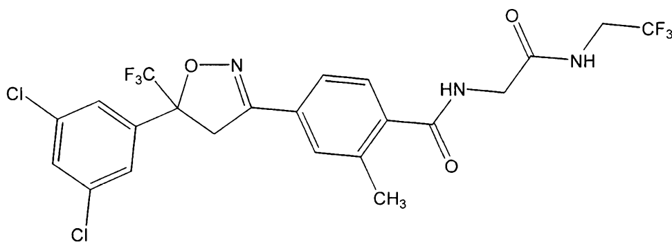
Fluralaner
