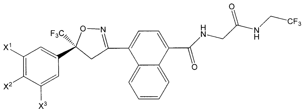
(S)-IA
