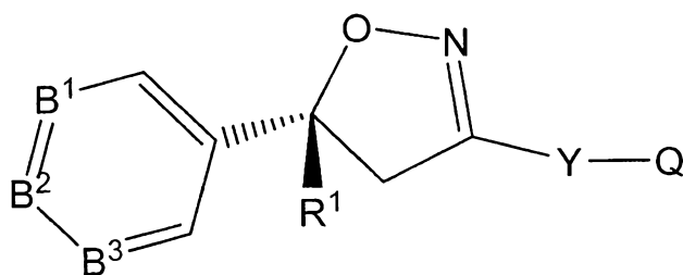
(R)-I
