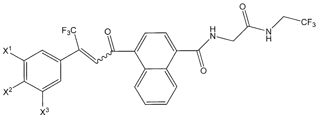
(IIA)
