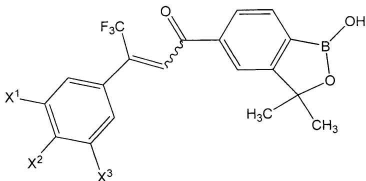
(IIE)
