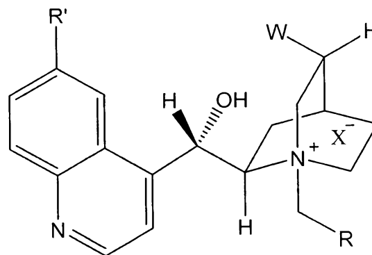
(IIIb)
