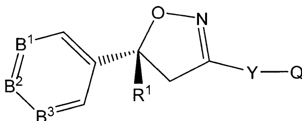
(R)-I
