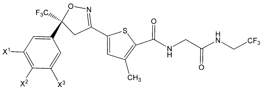
(S)-ID
