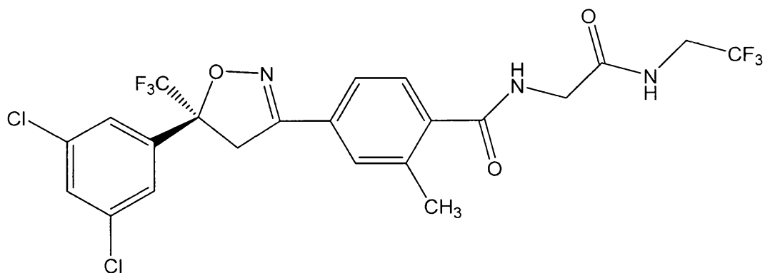
(S)-fluralaner
