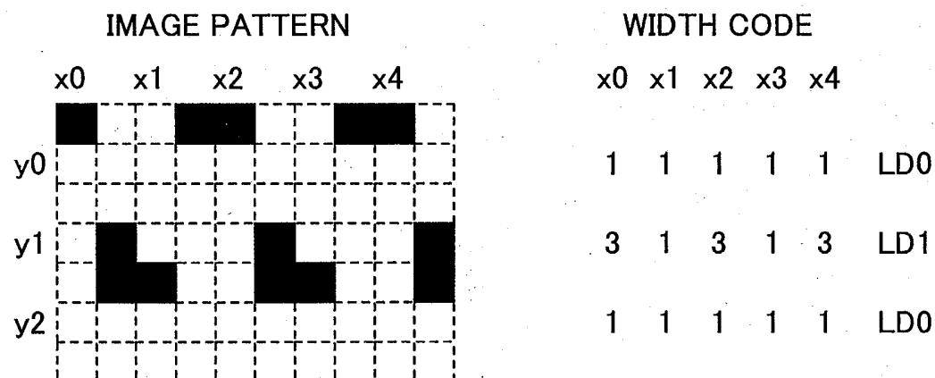
FIG.13E
