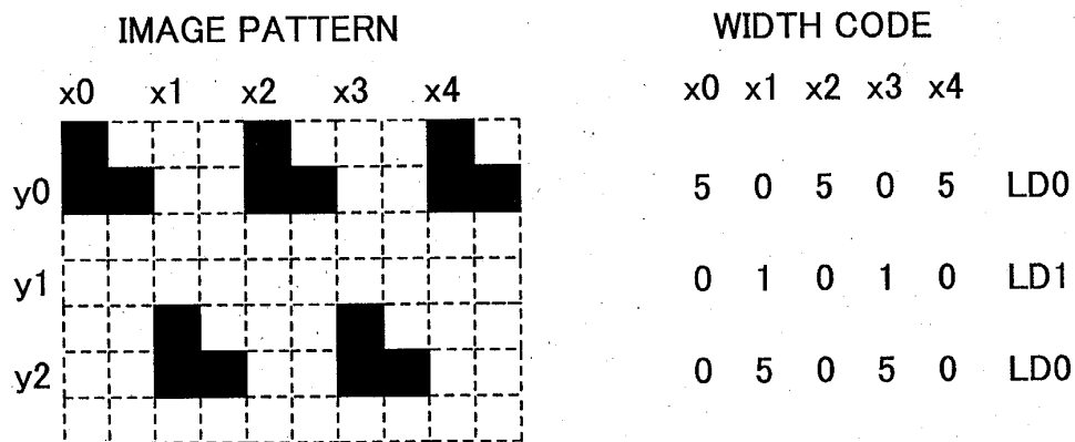
FIG.13B
