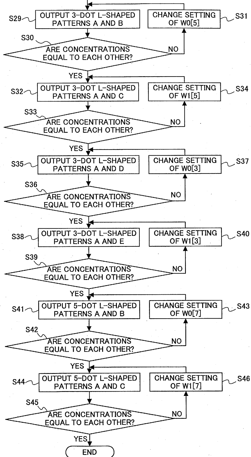
② FIG.17
