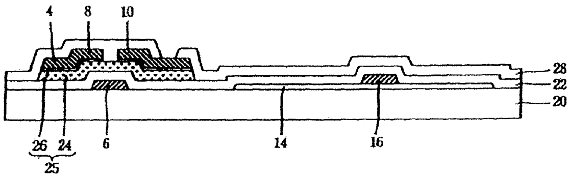
FIG. 2E RELATED ART
