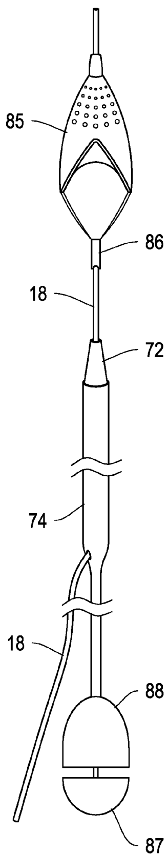
FIG. 8A
