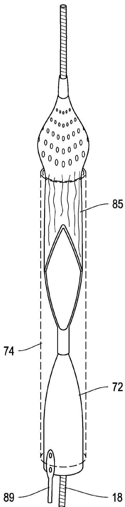
FIG. 9B
