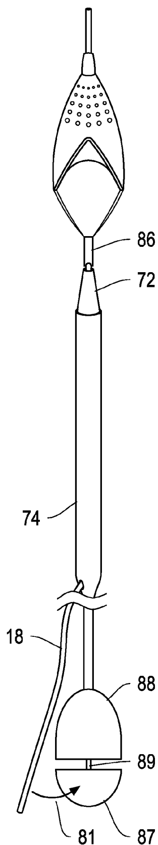
FIG. 8B
