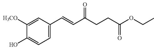
Monomer-7
