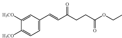
Monomer-5
