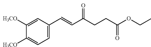
Monomer-6
