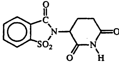
supidimide.
