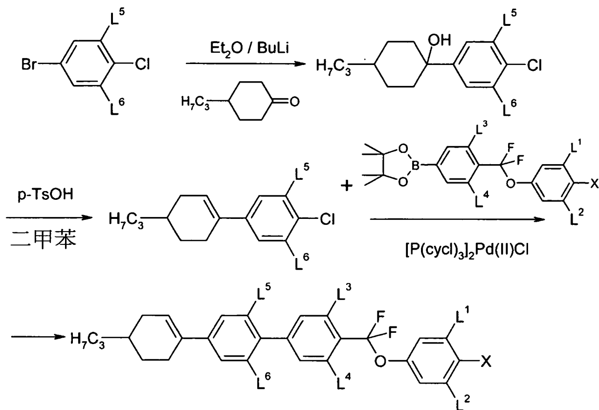
流程3：式I2化合物之合成。
