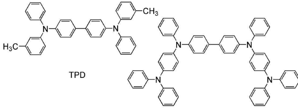
DPAB
