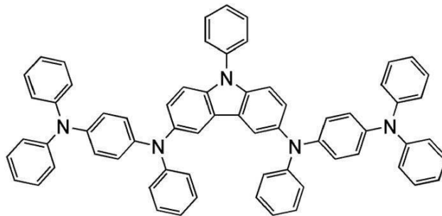
PCzDPA2
