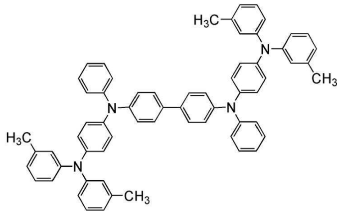
DNTPD
