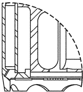
DETAIL E SCALE 2:1 FIG. 3B
