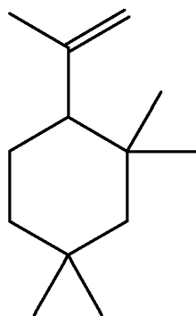
1-isopropenyl-2,2,4,4-tetramethylcyclohexane
