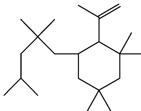
1-isopropenyl-2,2,4,4-tetramethyl-6-(2,2,4-trimethylpentyl)-cyclohexane
