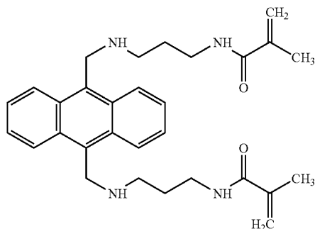
A. 9,10-bis[3-(methacrylamido)propylamino]methyl-anthracene
