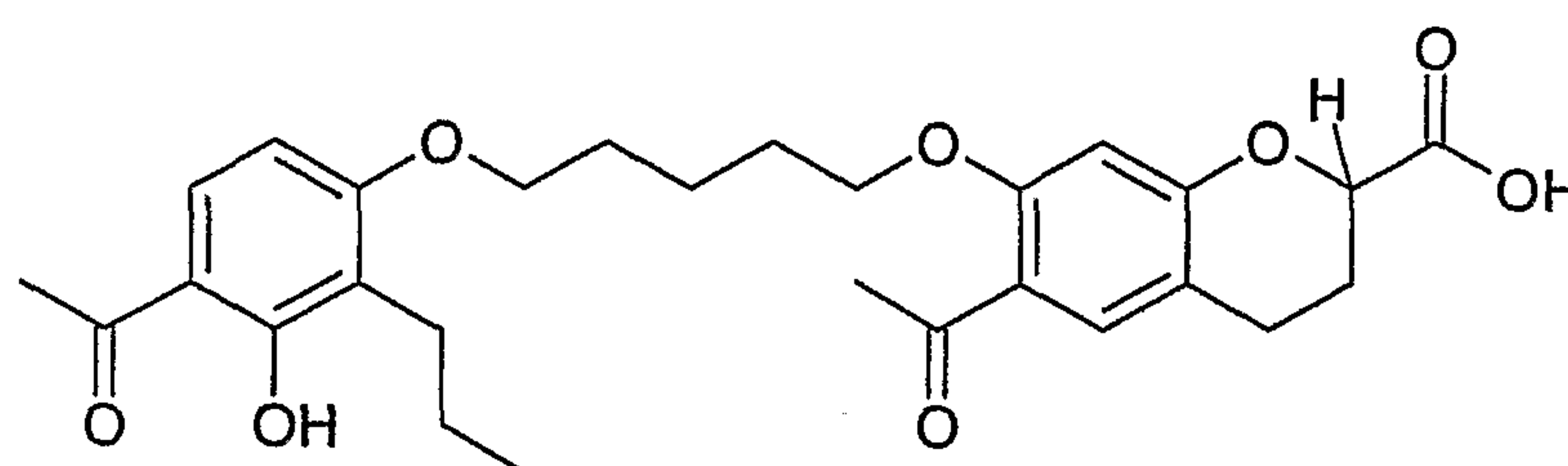
Ablukast
