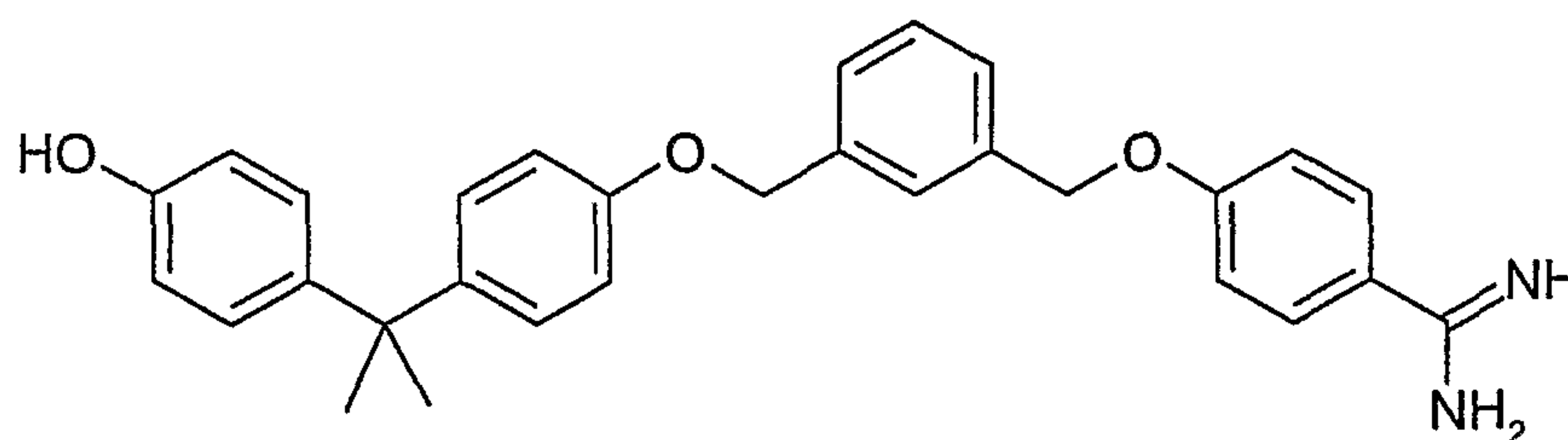
BIIL 284/260
