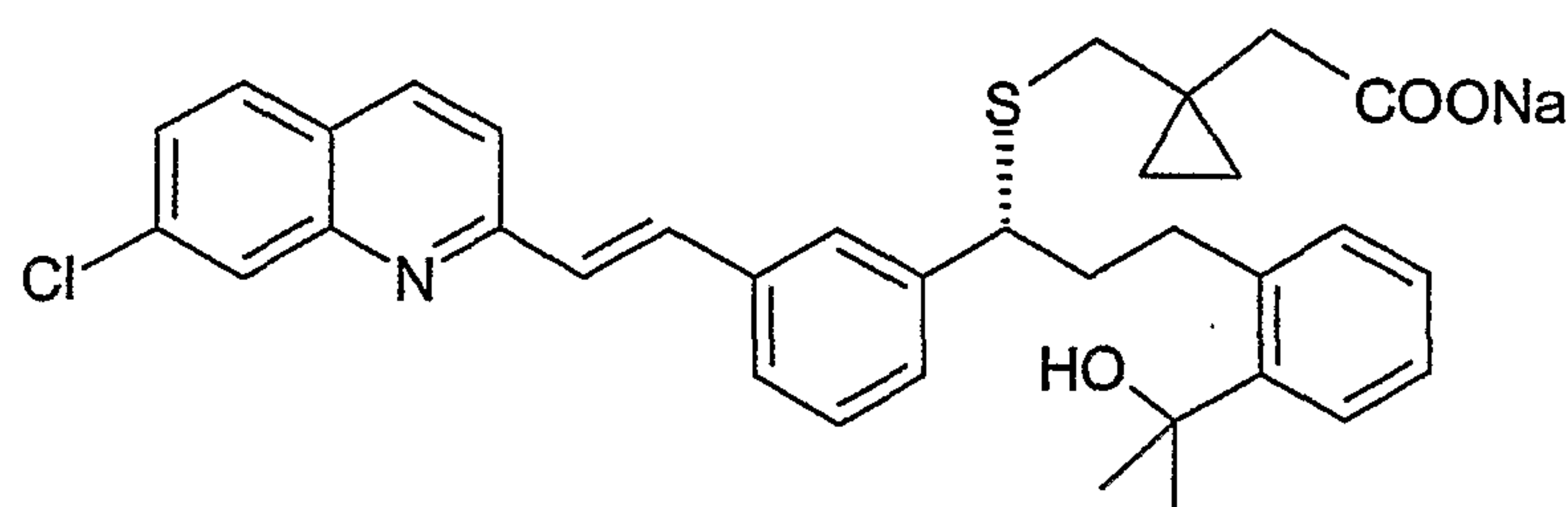
Montekulast
