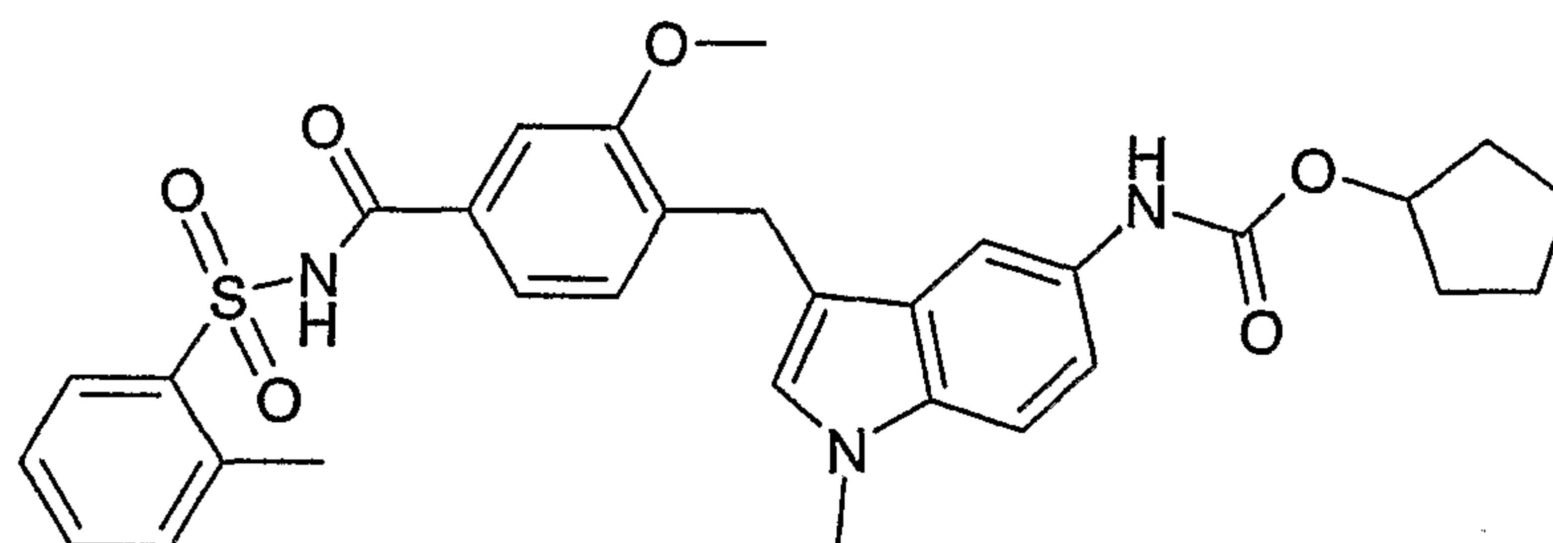
Zafirlukast
