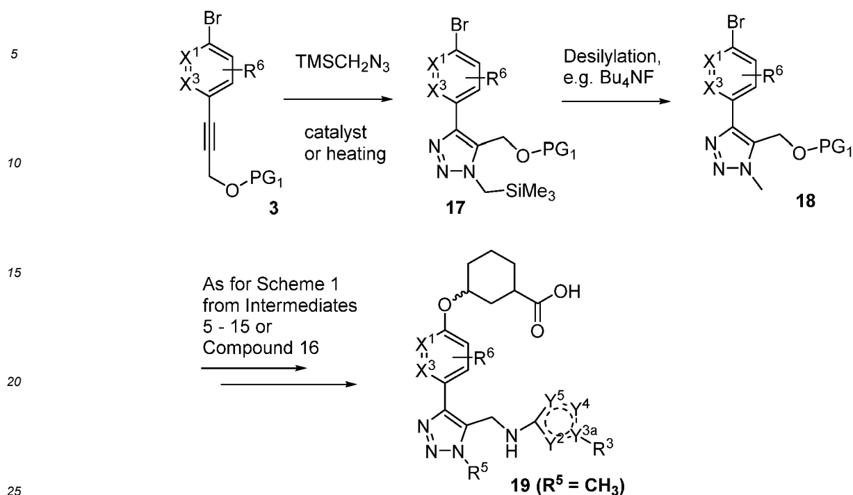
Scheme 1A
