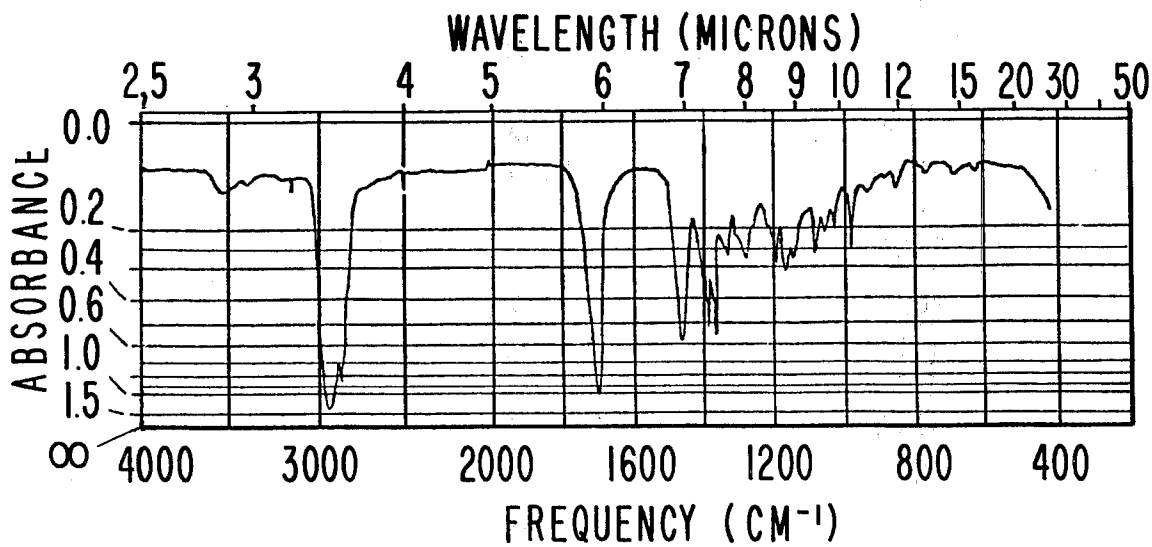
IR SPECTRUM
