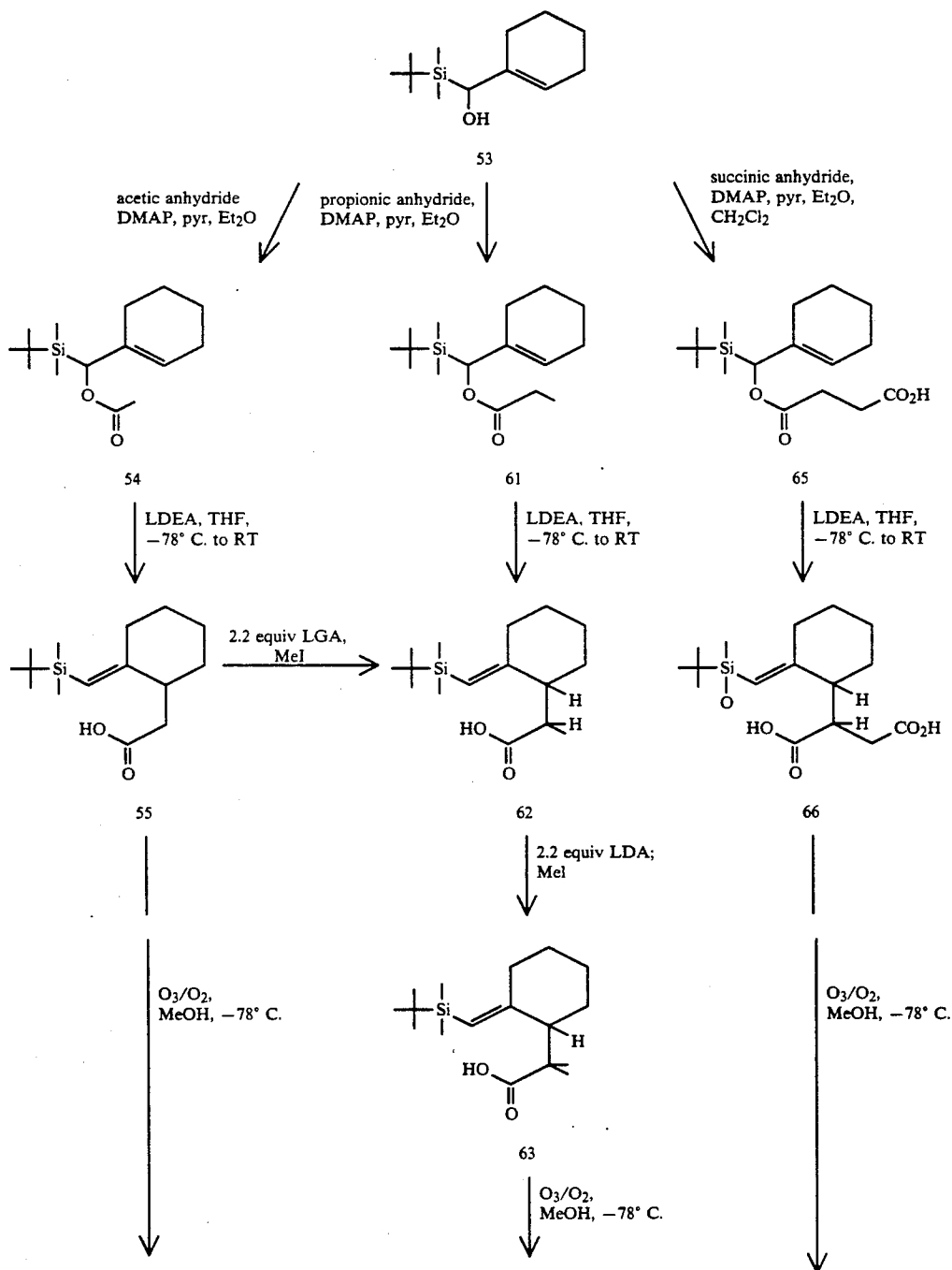
Scheme VI
